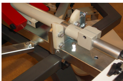
TEXIPRINT i utförande 6/6 med standard ramfäste Bild visar underredskonstruktionen för modell FPK.
